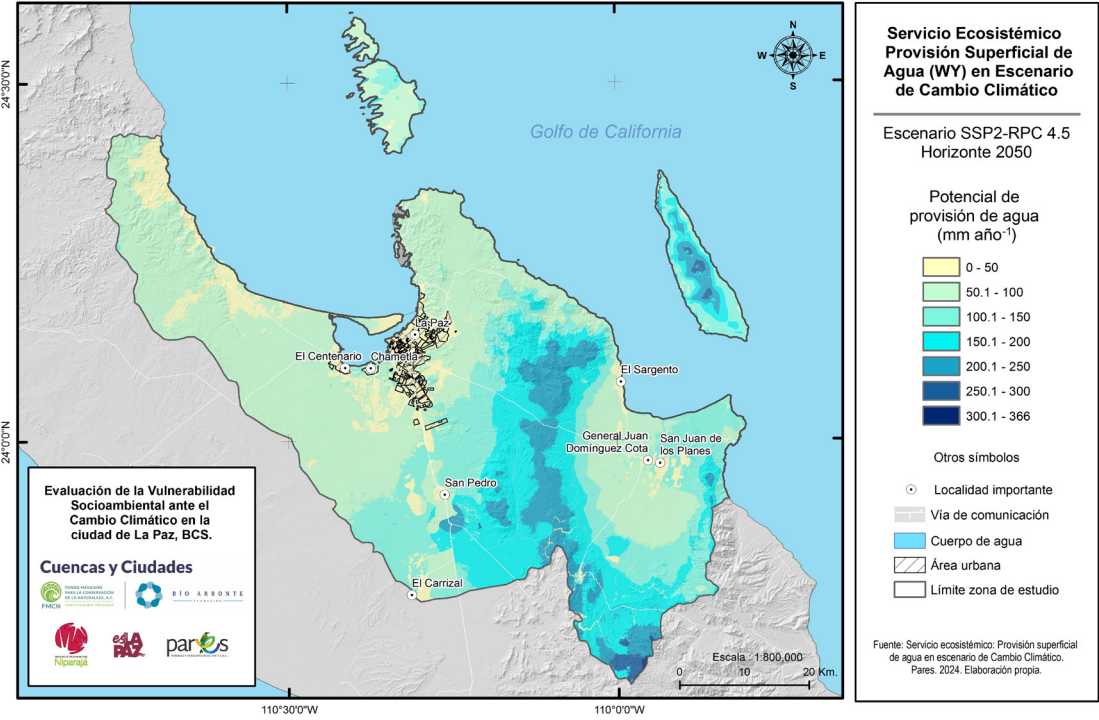
Figura 71. Provisión superficial del agua en escenario RCP 4.5 (2050). Fuente: Pares A.C.
