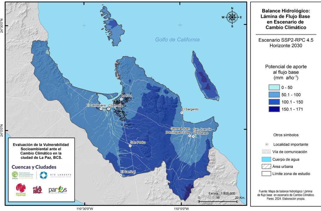
Figura 85. Aporte flujo base en escenario RCP 4.5. (2030). Fuente: Pares, A.C.
