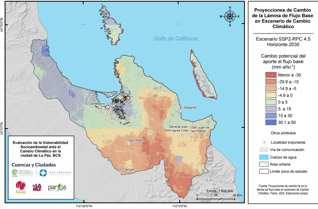
Figura 86. Cambio potencial en el flujo base en escenario RCP 4.5. (2030). Fuente: Pares, A.C.
