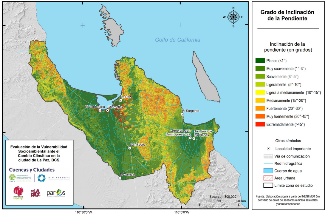
Figura 27. Grado de inclinación de la pendiente. Fuente: Pares A.C. con información de INEGI, 2015.
