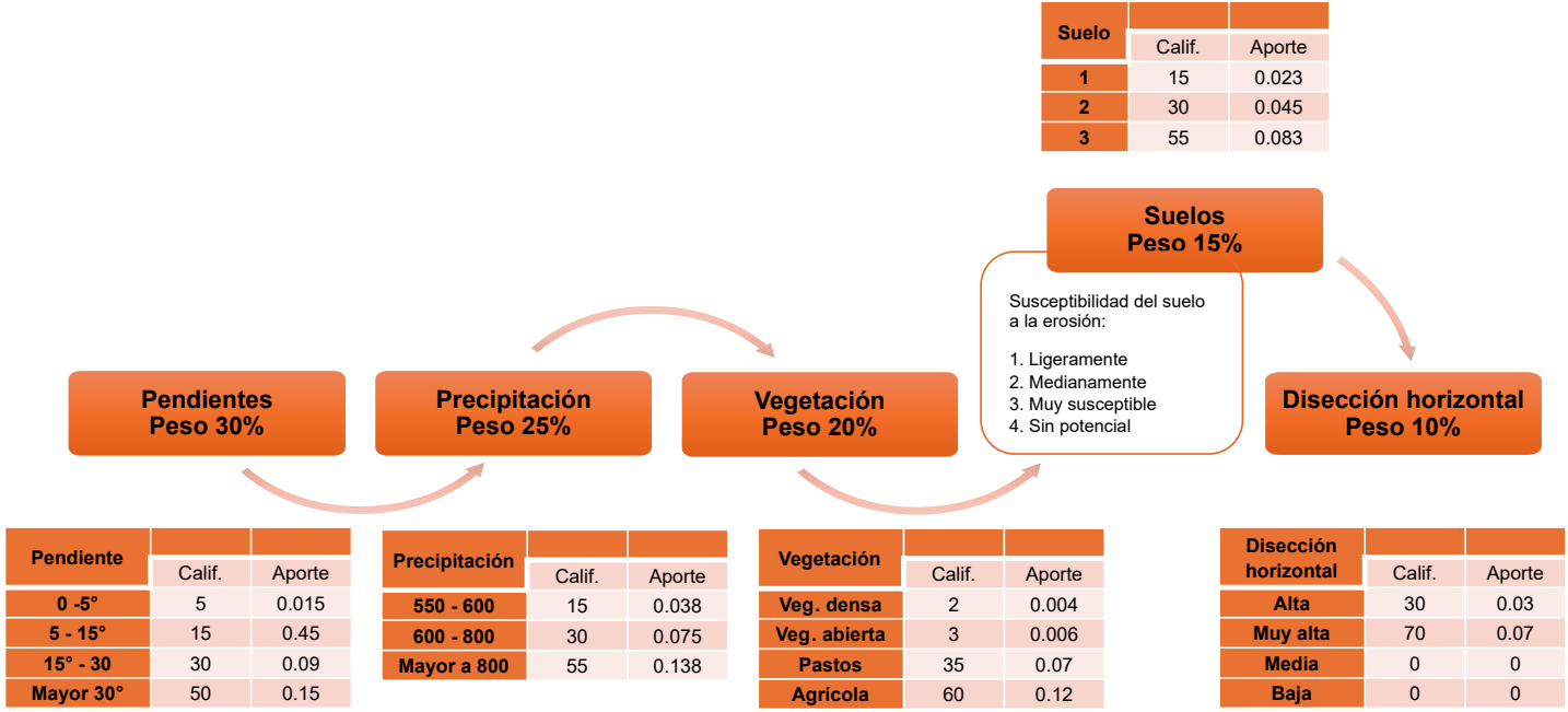
Figura 37. Modelo de potencial natural de erosión: variables y pesos ponderados. Fuente: Pares, A.C.
