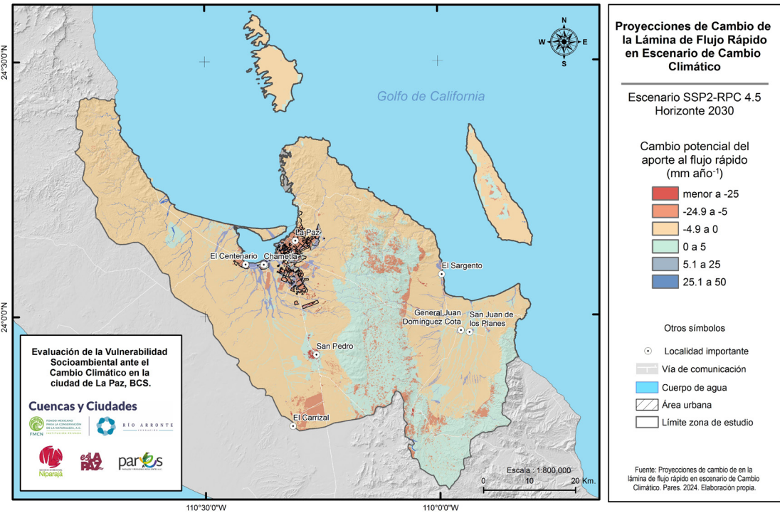
Figura 82. Cambios potenciales en el flujo rápido en escenario RCP 4.5. (2030). Fuente: Pares, A.C.
