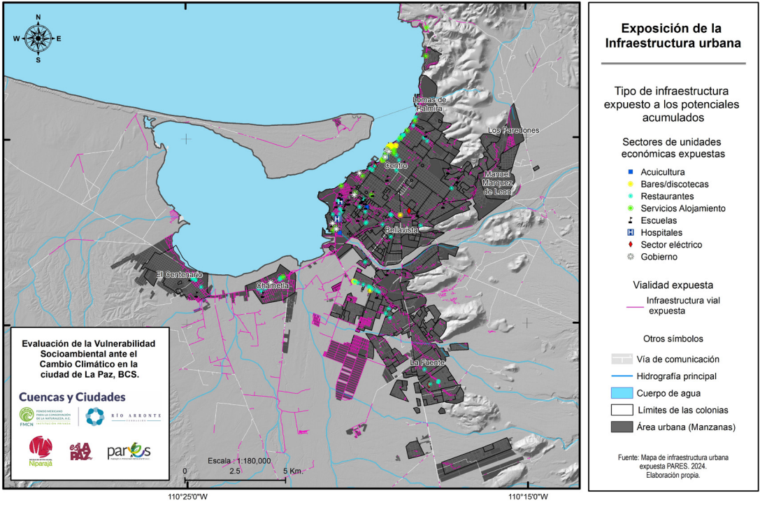
Figura 46. Exposición de la infraestructura urbana ante eventos climáticos. Fuente: Pares A.C.
