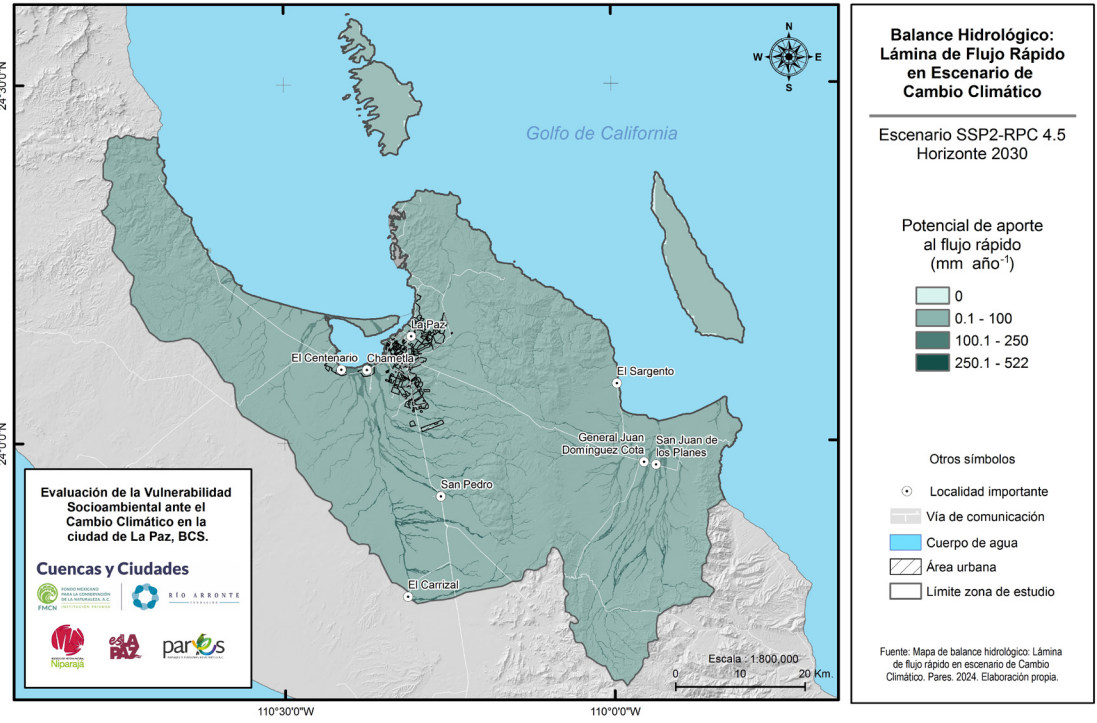
Figura 81. Potencial de aporte al flujo rápido en escenario RCP 4.5. (2030). Fuente: Pares A.C.
