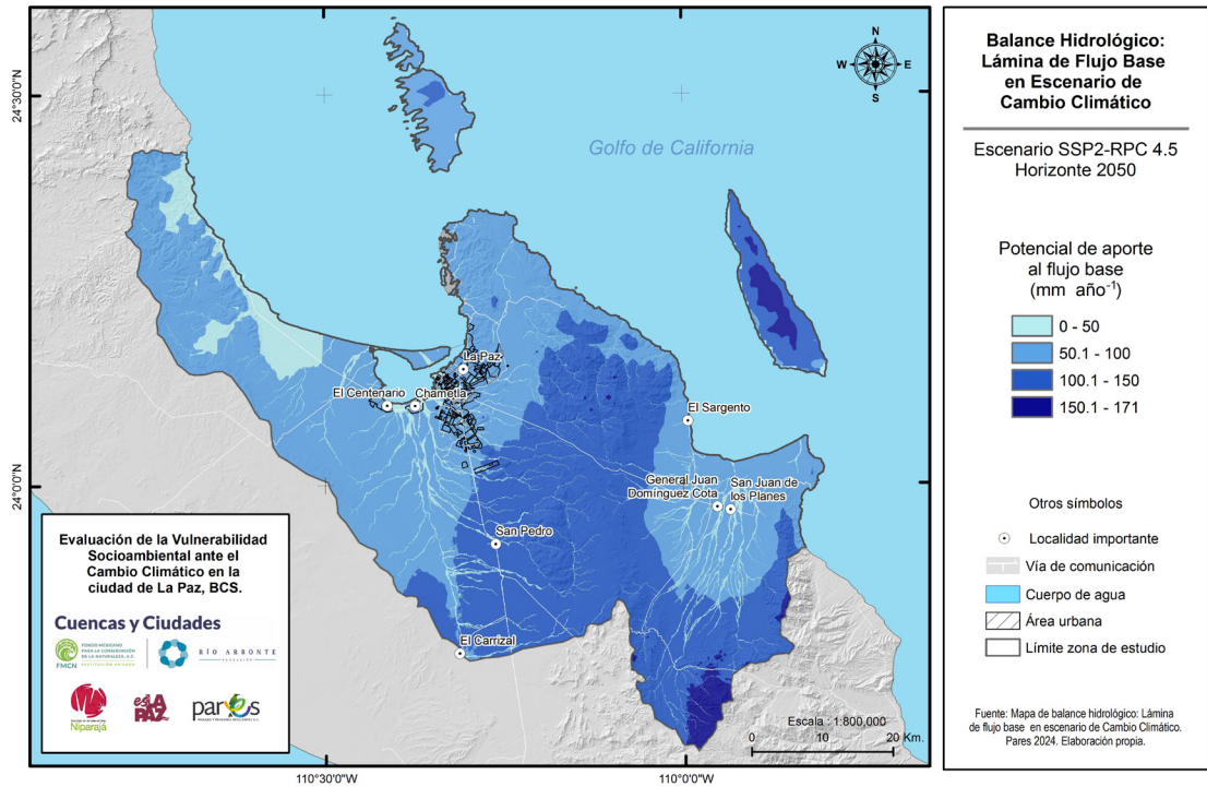
Figura 87. Aporte flujo base en escenario RCP 4.5. (2050).Fuente: Pares, A.C.
