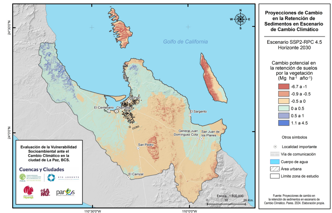
Figura 74. Cambios potenciales en la retención de sedimentos en escenario RCP 4.5 (2030). Fuente: Pares A.C.
