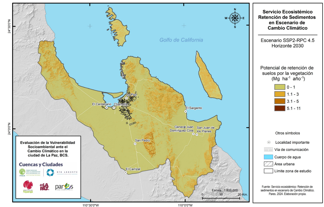
Figura 73. Retención de sedimentos en escenario RCP 4.5 (2030). Fuente: Pares A.C.
