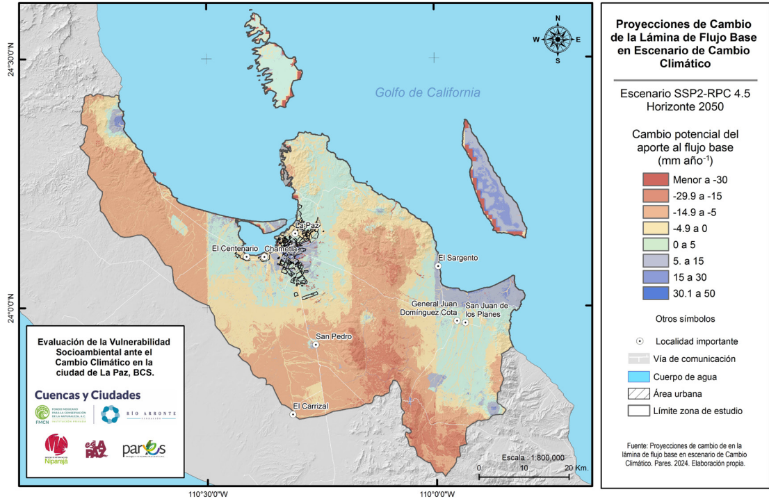
Figura 88. Cambio potencial en el flujo base en escenario RCP 4.5. (2050). Fuente: Pares, A.C.
