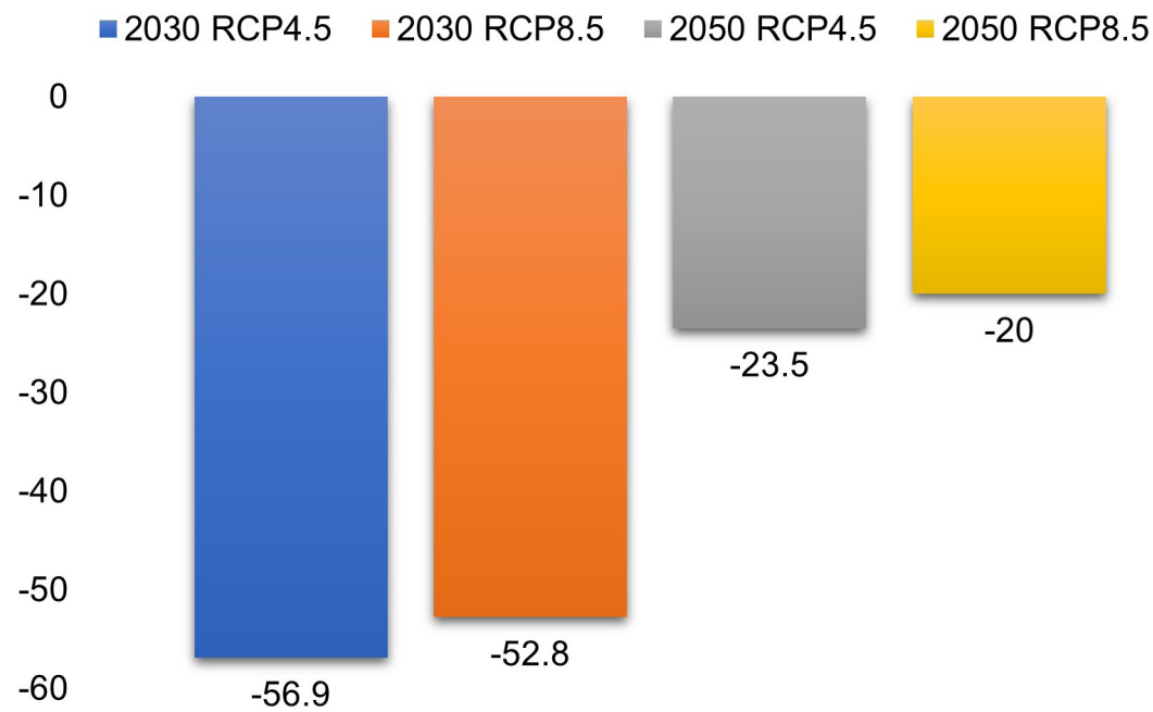
Gráfica 40. Cambios potenciales en la provisión superficial del agua en escenarios al 2030 y 2050 con RCP 4.5 y 8.5 (%). Fuente: Pares, A.C.
