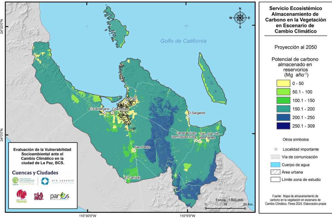
Figura 79. Almacenamiento de carbono en escenario RCP 4.5. (2050). Fuente: Pares A.C.
