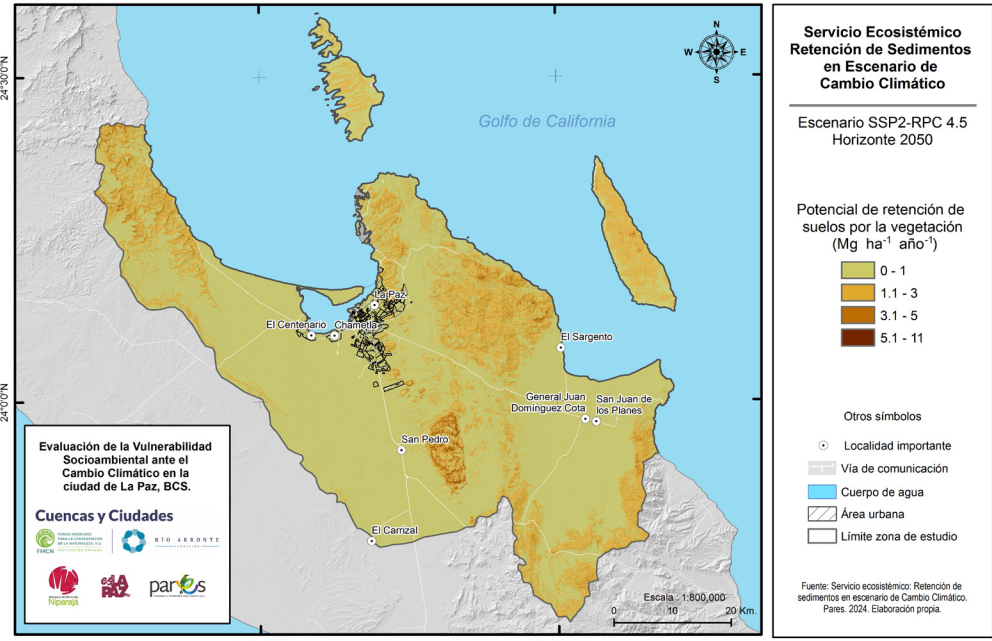
Figura 75. Retención de sedimentos en escenario RCP 4.5 (2050). Fuente: Pares, A.C.
