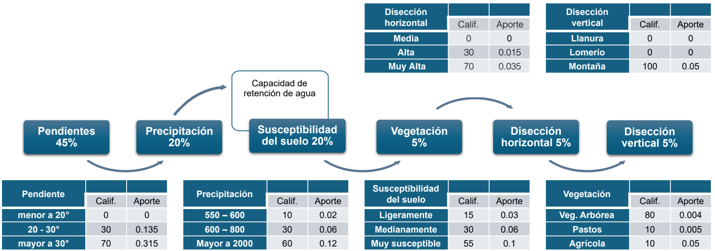
Figura 30. Modelo de potencial natural de deslizamientos: variables y peso ponderado. Fuente: Pares, A.C.
